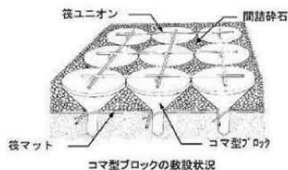
コマ型ブロックの敷設状況
