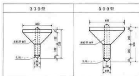
コマ型ブロックの断面寸法(単位:mm)
