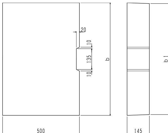
■形状図
