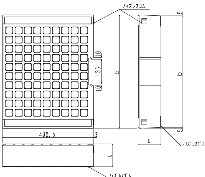
■形状図
