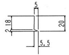
目地詳細図
