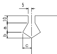
◆目地詳細図
