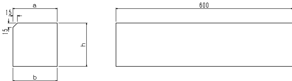
地先境界ブロック
