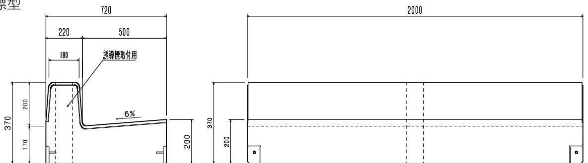
路面排水柵用型(2分割)
