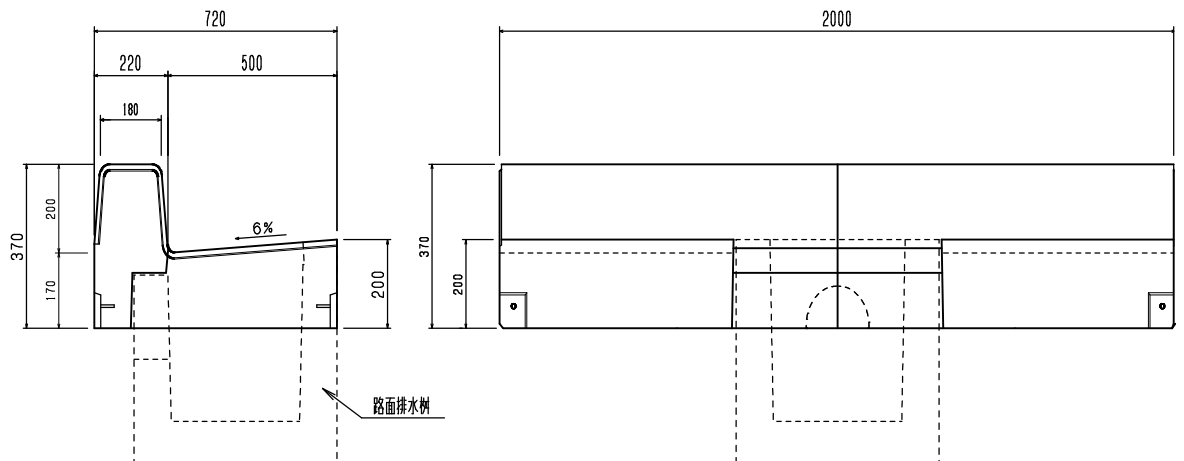
路面排水柵用型(2分割)
